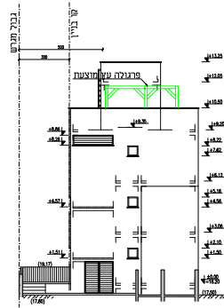
חזית צפונית ק.מ. 1:100
