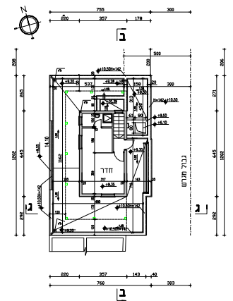
תוכנית גגות ק.מ. 1:100
