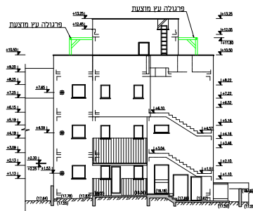
חזית מזרחית ק.מ. 1:100
