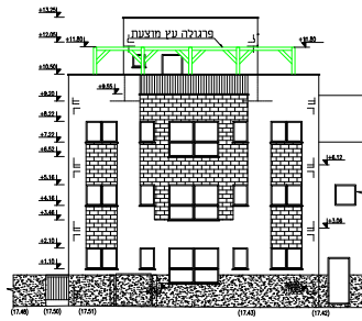
חזית מערבית ק.מ. 1:100
