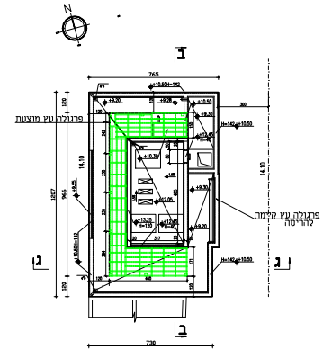
תוכנית גג עליון ק.מ. 1:100
